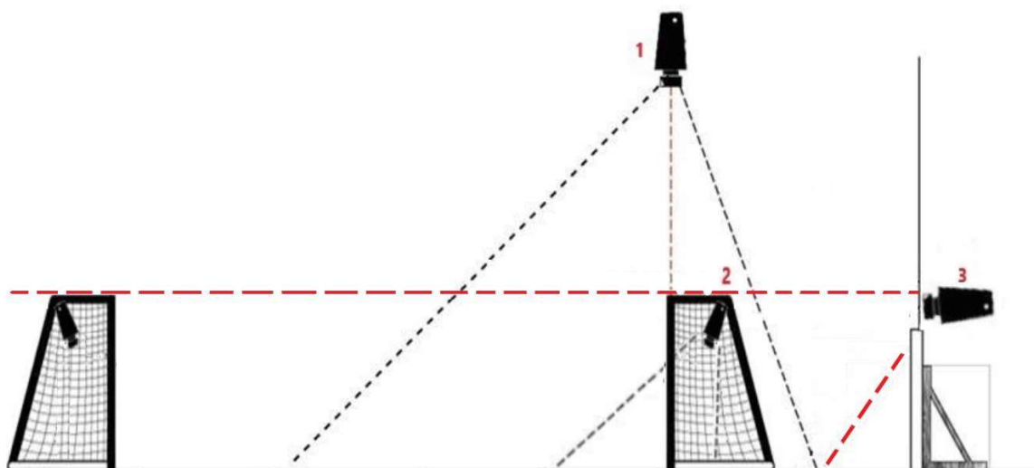
Схема расположения камер над воротами и за воротами (вид сбоку)
