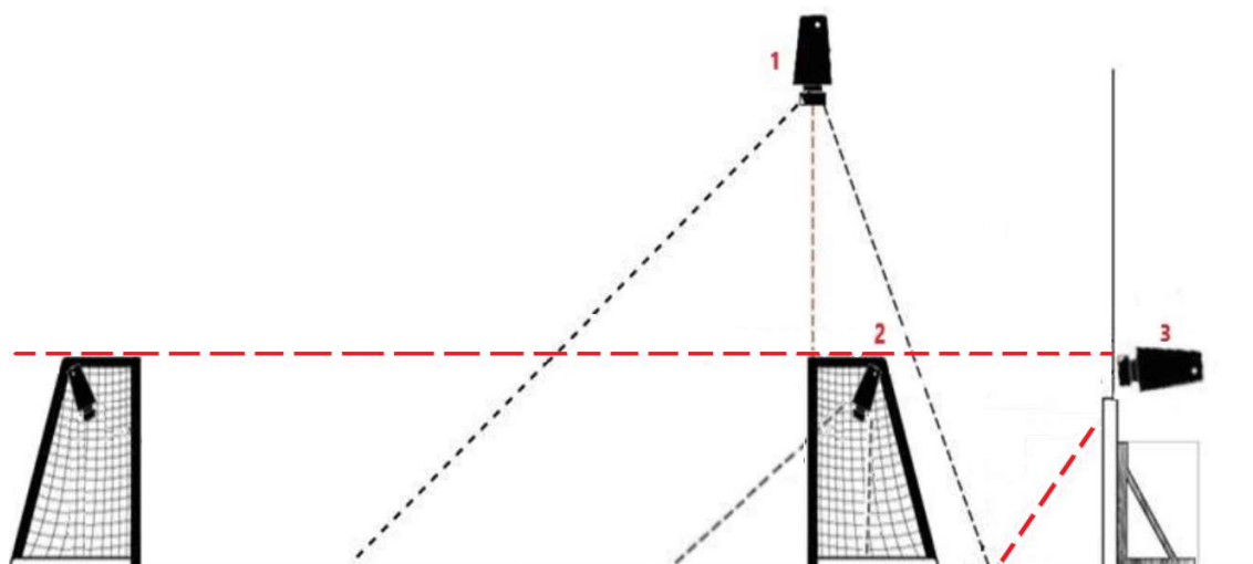
Схема расположения камер в воротах, над воротами и за воротами (вид сбоку)
